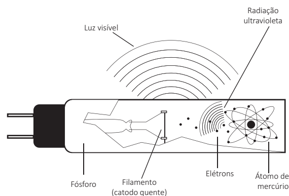
Figura 3 – Funcionamento da lâmpada fluorescente
